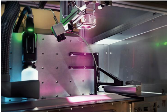
Bild 1: Trocknung mit Diodenlaser: Durch die spezielle Optik bestrahlt der Laser eine größere Fläche auf der mit Graphitpaste beschichteten Kupferfolie. Die Wechselwirkung der Graphitpartikel mit der Lichtenergie erzeugt Wärme, und die Flüssigkeit ver- dampft. © Fraunhofer ILT, Aachen.
